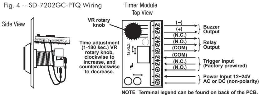
Fig. 4 -- SD-7202GC-PTQ Wiring
